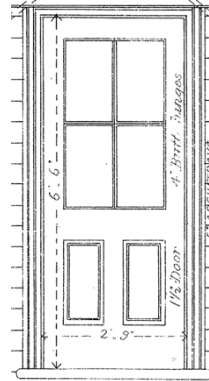
Door Gatekeepers Cottage
