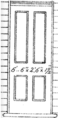
Door Gatekeepers Cottage 6' 6" x 2' 6" x 1 1/2"
